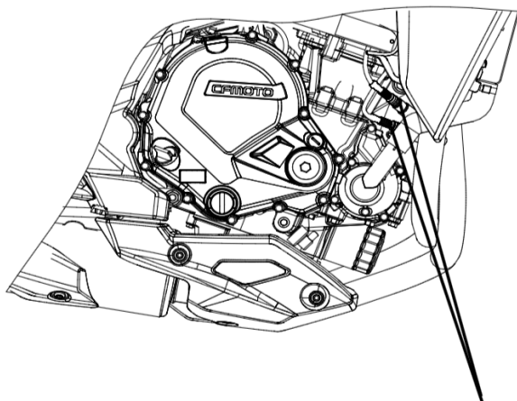
Kyslíkové čidlo
