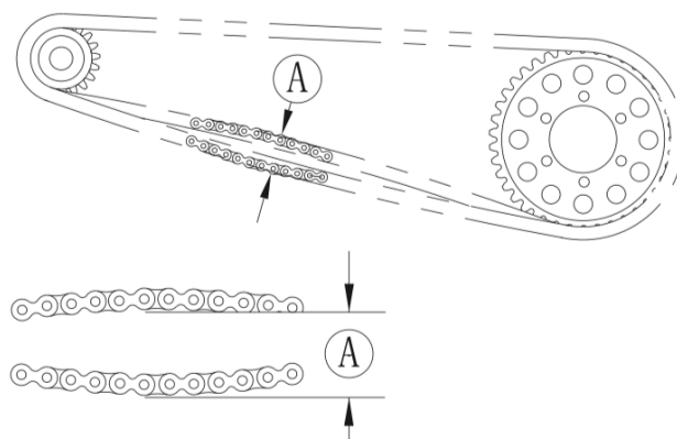
Ⓐ Povolení řetězu
